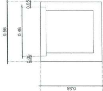
รูปด้านรางระบายน้ำ
